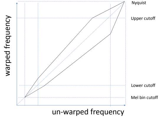
Fig. 1. VTLN warping function
